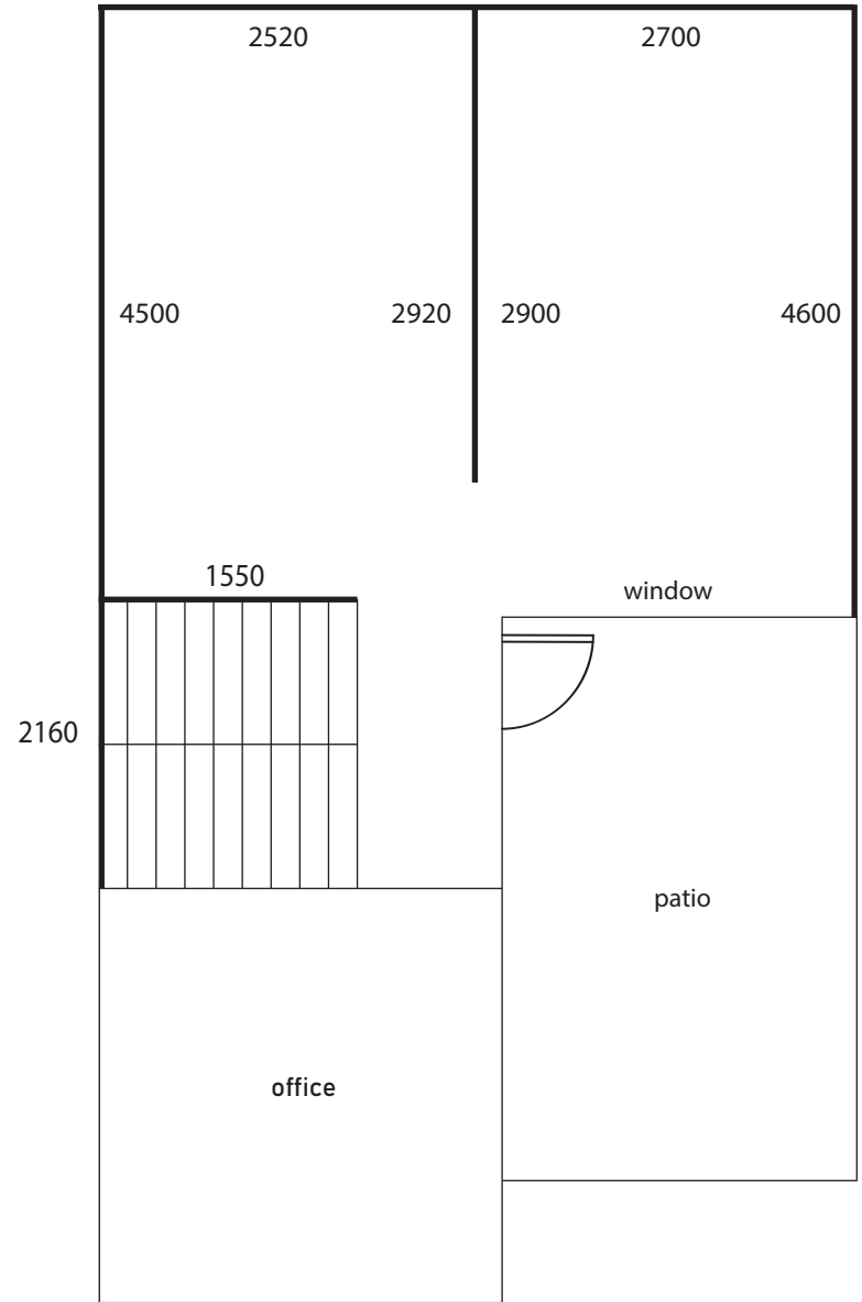
2F Height 2750
